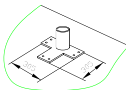
Variante B: Soporte atornillado
