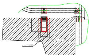
Variante A: Soporte empotrado
